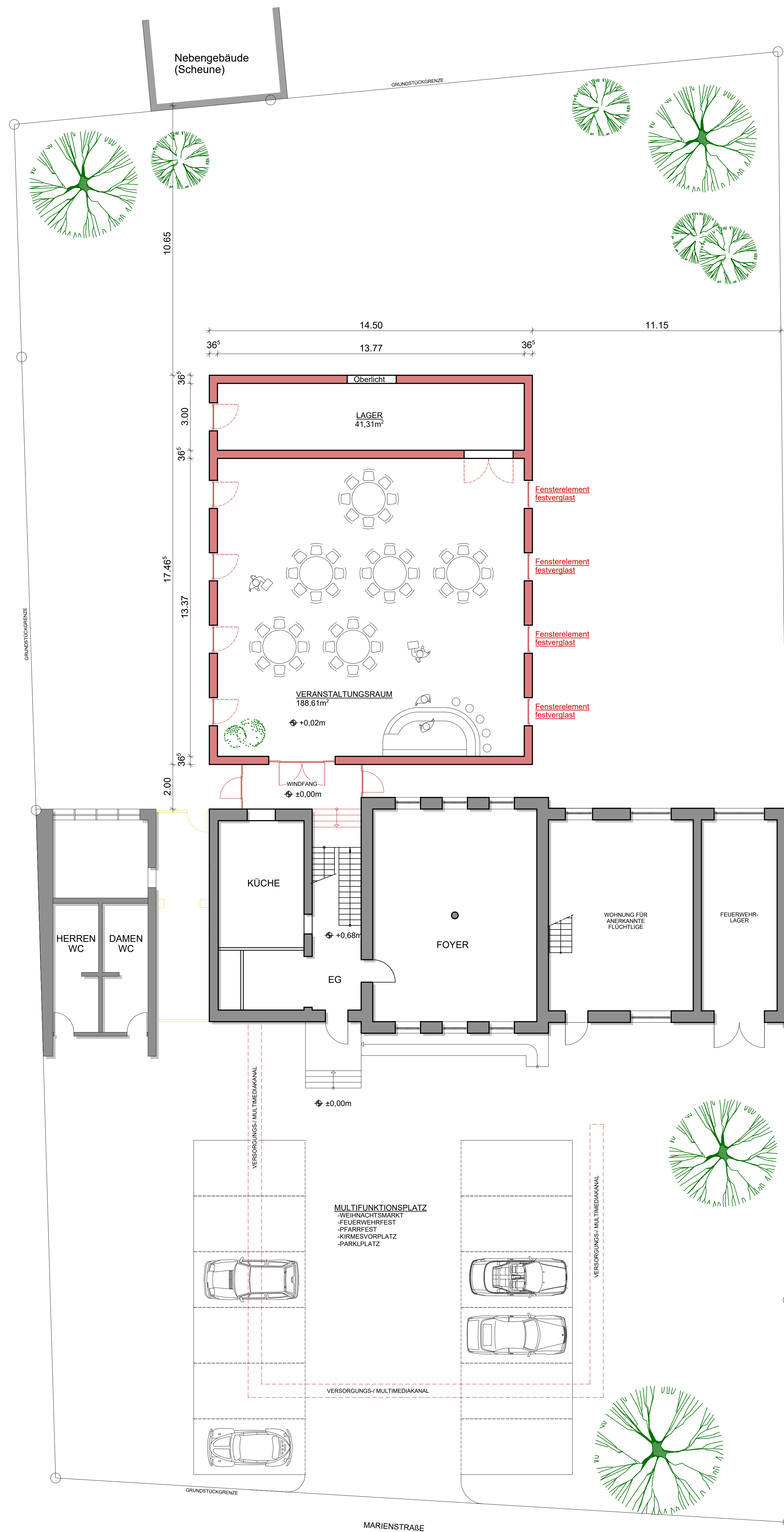
DRAUFSICHT ERDGESCHOSS
